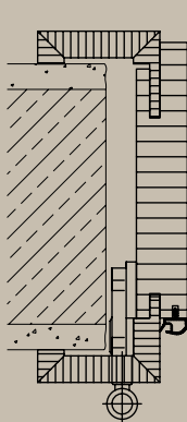
Dřevěná zárubeň, ostrá hrana
