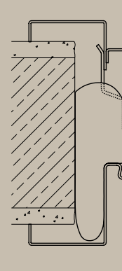
Ocelová zárubeň VarioFix
